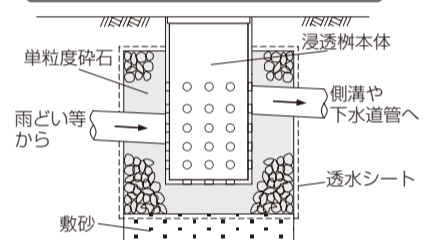
雨水浸透施設(浸透柵)の設置例
