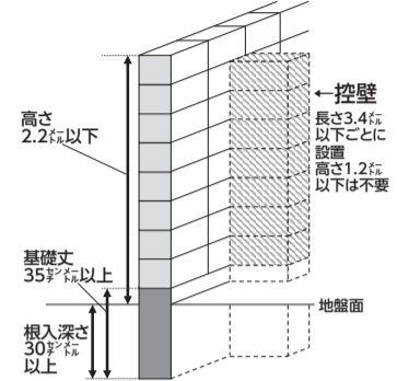
図1:外観から分かるブロック塀の規定
