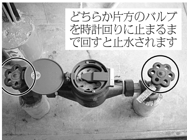
止水栓 (集合住宅)
