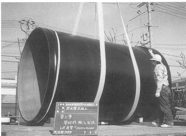
飲料水兼用型貯水槽の搬入状況（今津中学校）
