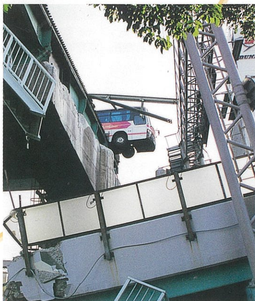
落橋した阪神高速・神戸線上で間一髪、転落を免れた長距離スキーバス (本町付近)
