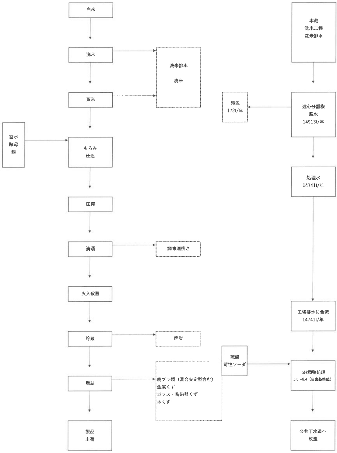
図2 洗米排水処理フローシート
