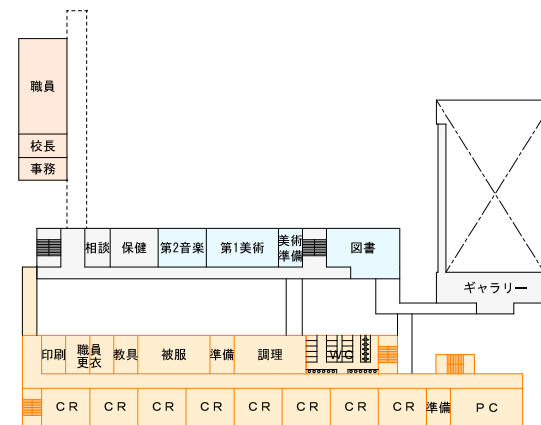
2階平面図 1/1000
