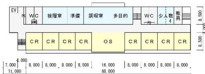
4階平面図
