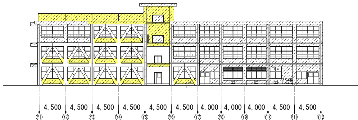
東校舎 東側立面図
