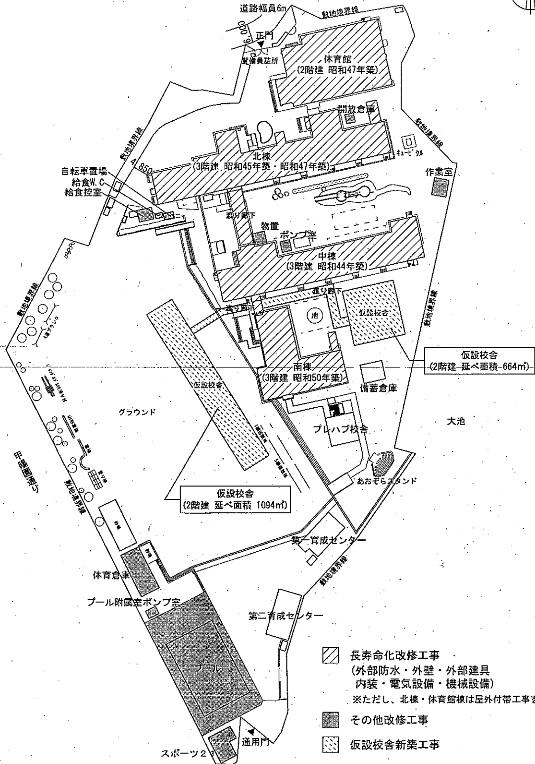
甲陽園小学校長寿命化改修他工事 配置図 (1/1200)
