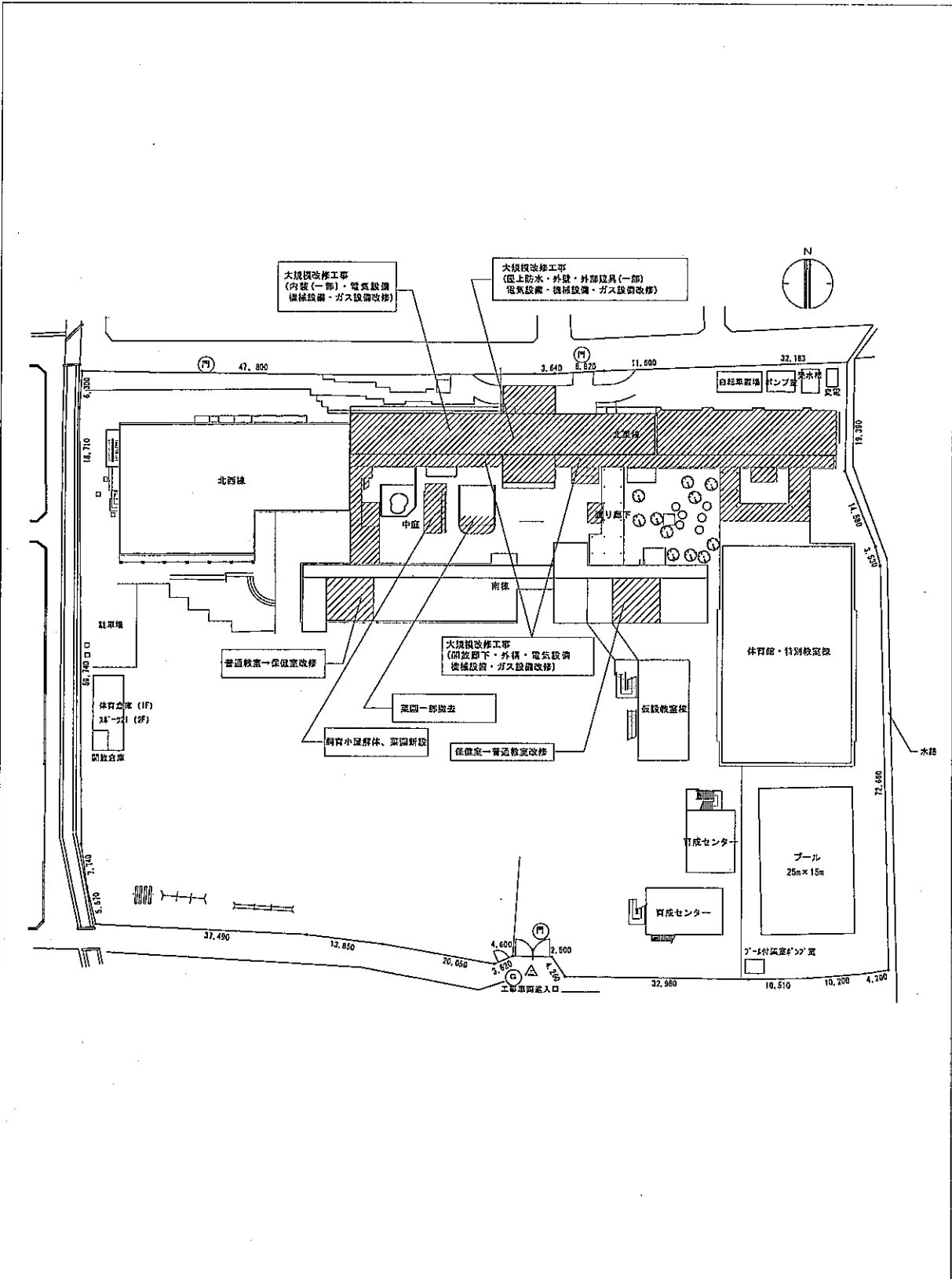
甲東小学校北東棟大規模改修工事 配置図(1/1000)
